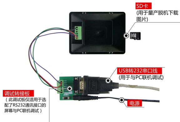
图 1-4 RS232 调试工具图
