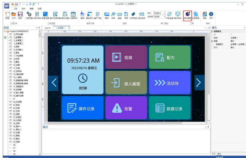
图 10-1LUA 脚本编程
