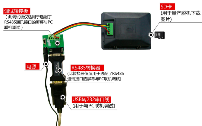
图 1-5 RS485 调试工具图
